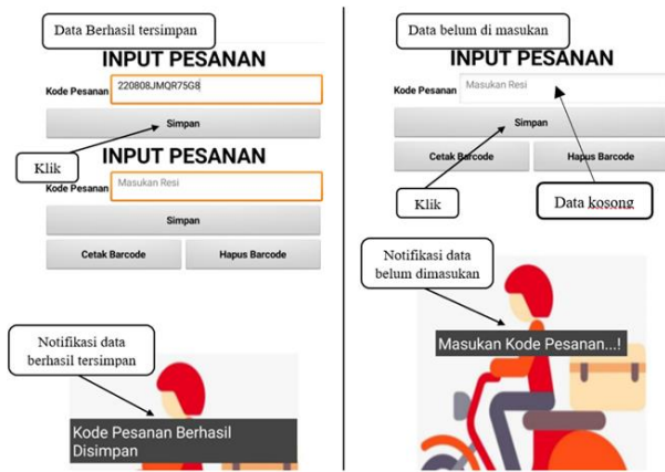
Gbr. 12 Cara Kerja Button Simpan
