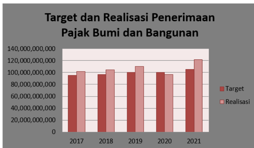
Gambar 2. Grafik Penerimaan PBB
