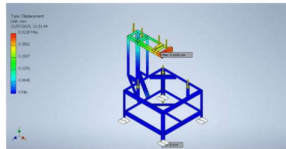
Gambar 5. Hasil Perpindahan
