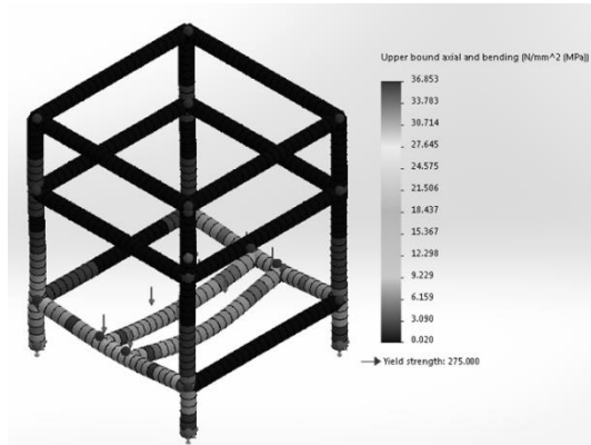
Gambar 2. Hasil uji kekuatan rangka terhadap beban menggunakan solidwork
