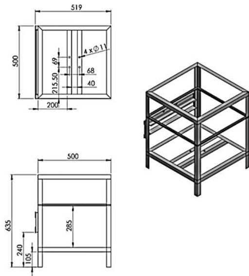
Gambar 1. Desain Rangka
