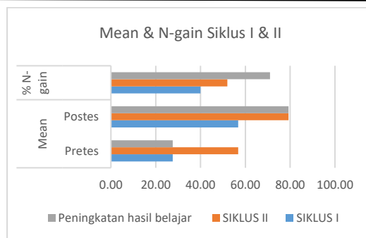
Gambar 3. Grafik Mean dan N-gain Pretes-postes untuk 2 Siklus
