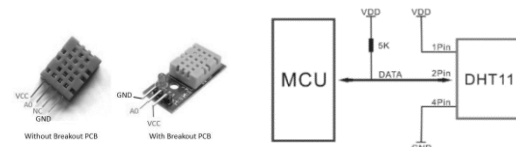
Gambar 7. Sensor suhu dan kelembaban DHT11 (Syam, 2013)
