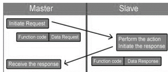
Gambar 5. Konsep dasar MODBUS RTU (CIMON CO., 2015)
