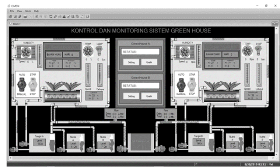
Gambar 21. SCADA CIMON
