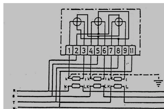
Gambar 2.1 Pengawatan kVArh meter tiga fasa[12].
