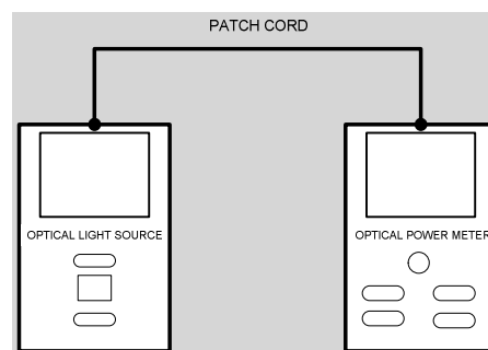
Gambar 12 Kalibrasi OPM
