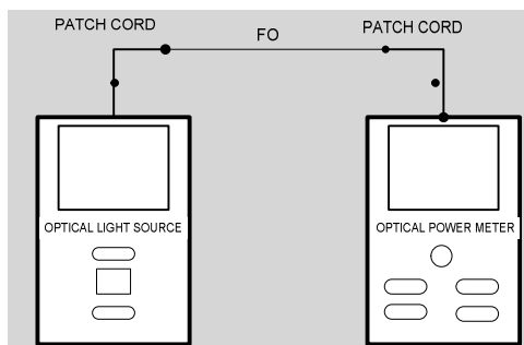
Gambar 13 Pengukuran Redaman Kabel dengan OPM
