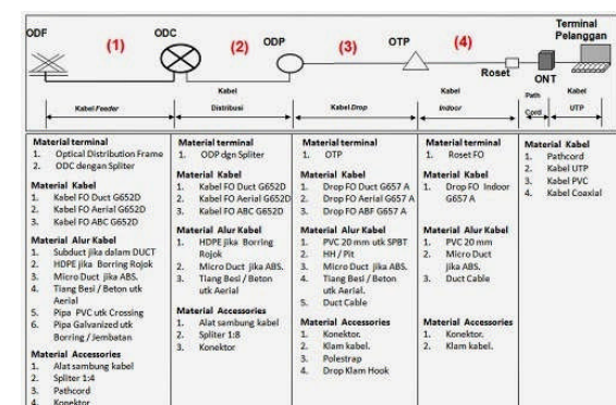
Gambar 1 Konfigurasi FTTH & List Material
