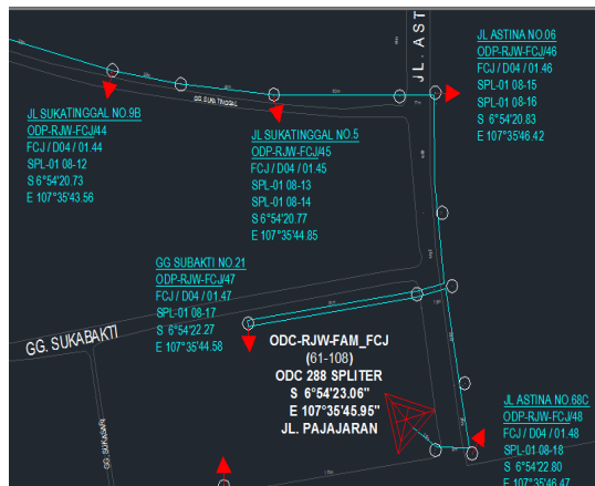
Gambar 18 Peta Lokasi ODC & ODP
