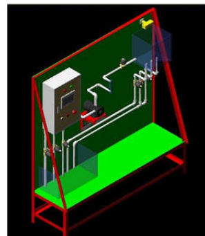
Gambar 6. Desain sistem keseluruhan
