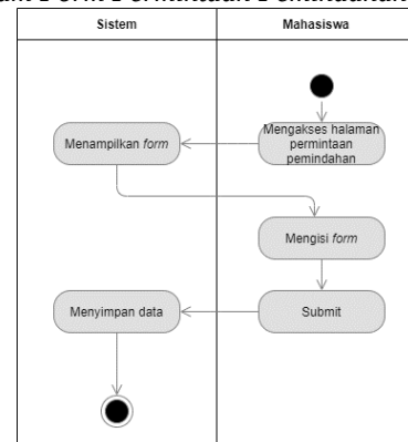
Gbr 10. Activity Diagram Form Permintaan Pemindahan
