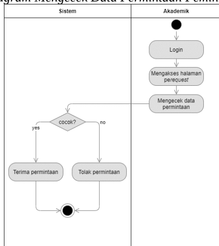
Gbr 7. Activity Diagram Mengecek Data Permintaan Pemindahan
