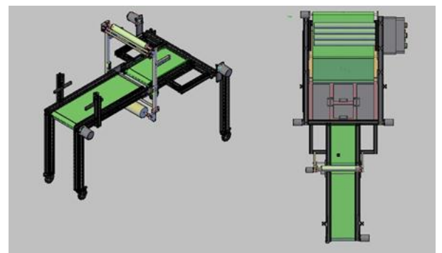
Gbr.3 Hasil Desain Alat
