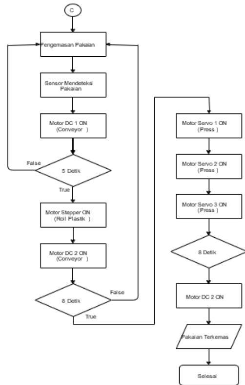
Gbr. 2 Flowchart Pengemasan
