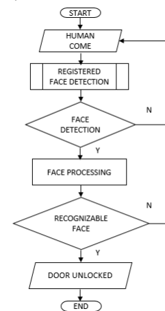
Gbr. 4 Diagram Alir Proses Pengujian
