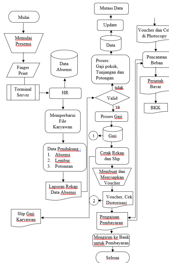
Gambar 1. Flowchart Sistem Informasi Penggajian pada PT. Kertas Padalarang
